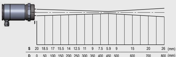
CF4 optics 75:1
