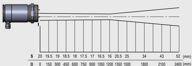
SF optics 75:1
