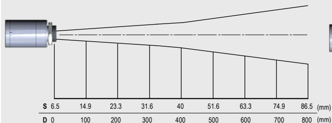
10:1 optics
